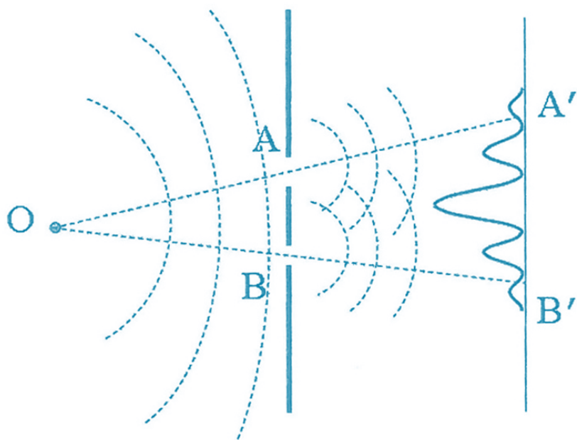
Σχ. 3. Κροσσοί συμβολής των φωτεινών κυμάτων από την πηγή O που διέρχονται από τις όπες A και B και παρατηρούνται στο πέτασμα A'B' .
