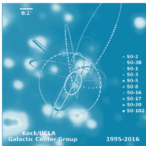
Σχ. 1. Τροχιές γύρω από τη μελανή όπη στο Κέντρο του Γαλαξίου.
