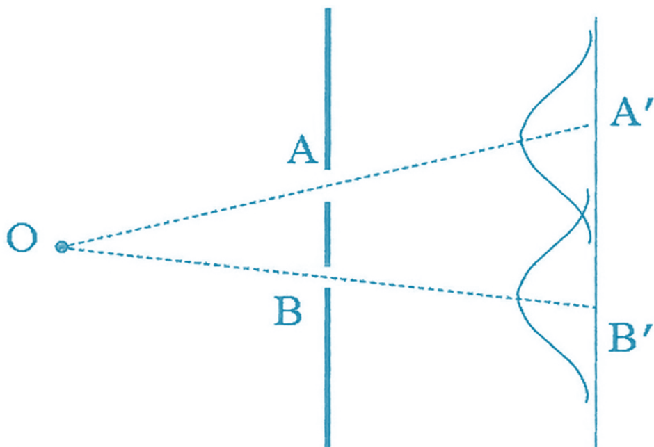
Σχ. 2. Τροχιές (κλασικών) βλημάτων από την πηγή O δια μέσου των όπων A και B και κατανομή των βλημάτων στο πέτασμα A'B' .
