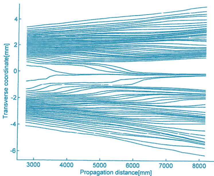
Σχ. 5. Τροχιές τύπου Bohr στα πειράματα των Kocsis et al. (2011).
