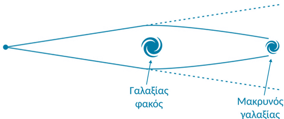
Σχ. 6. Βαρυτικοί φακοί.
