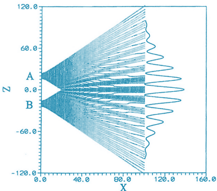
Σχ. 4. Κυματοειδείς τροχιές ηλεκτρονίων στη μηχανική του Bohr, που συμβάλλουν μετά τη διόδο τους από τις όπες A και B και δημιουργούν κροσσούς συμβολής.
