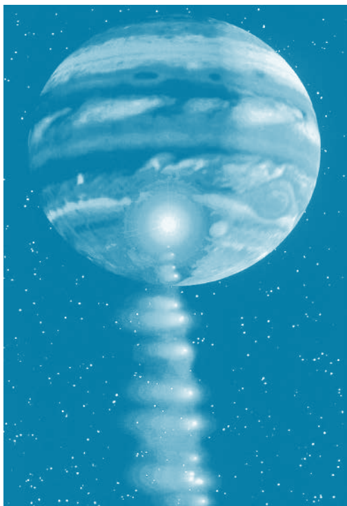
Ο κομήτης Σουμέικερ – Λέβη πέφτει πάνω στον Δία
