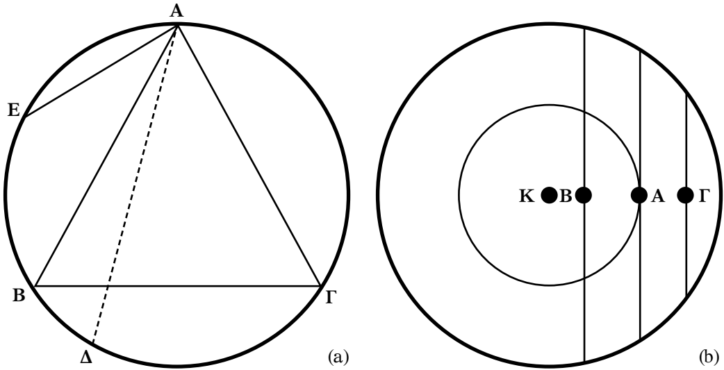
Σχήμα 1: (a) Η χορδή AD είναι μεγαλύτερη από την πλευρά του εγγεγραμμένου ισόπλευρου τριγώνου AB\Gamma , ενώ η χορδή AE είναι μικρότερη. (b) Η χορδή με κέντρο το A σε απόσταση KA = 1/2 της ακτίνας του κύκλου είναι ίση με την πλευρά ισόπλευρου τριγώνου, η χορδή με κέντρο το B είναι μεγαλύτερη και η χορδή με κέντρο το \Gamma είναι μικρότερη.
