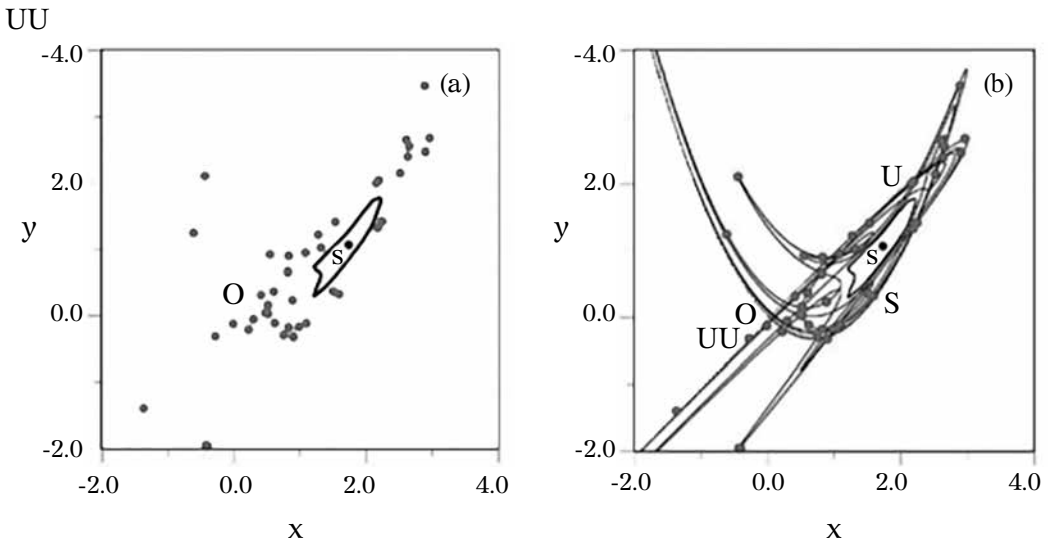
Σχήμα 5: (a) Τα διαδοχικά σημεία (x, y) μιᾶς τροχιάς φαίνονται τυχαία. (b) Όμως τα σημεία αυτά διατάσσονται πάνω σὲ μιὰ ἀσυμπτωτική καμπύλη U ἀπὸ τὴν ἀρχὴ τῶν ἀξόνων, ἡ ὁποία ἔχει πολλὲς ἀναδιπλώσεις (ἀπὸ τὸ σημείο O ἀρχίζουν 2 ἀσταθεῖς ἀσυμπτωτικὲς καμπύλες, U καὶ UU , καὶ δύο εὐσταθεῖς ἀσυμπτωτικὲς καμπύλες ( S καὶ SS )).
