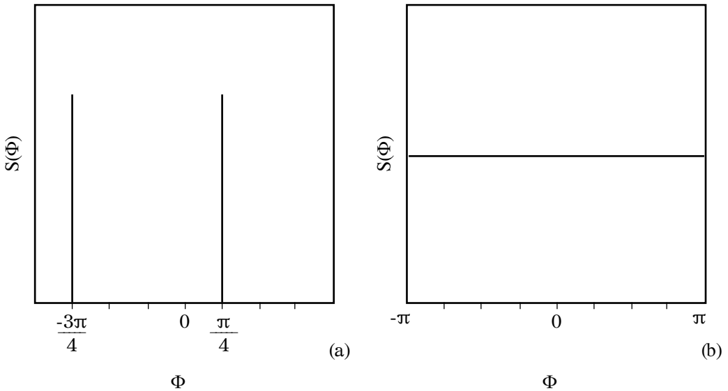
Σχήμα 4: (a) Τò φάσμα τῶν γωνιῶν ἐλικώσεως, ὅταν ἡ παράμετρος K τείνει στοῦ ἄπειρου, καὶ (b) τὸ φάσμα μιᾶς τυχαίας κατανομῆς.
