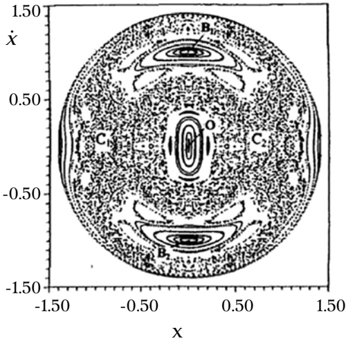
Σχήμα 3: Οί καμπύλες σε μιὰ επιφάνεια τομής Poincaré αντιπροσωπεύουν οργανωμένες τροχιές, ενώ τὰ διάσπαρτα σημεία αντιπροσωπεύουν χαοτικές τροχιές.
