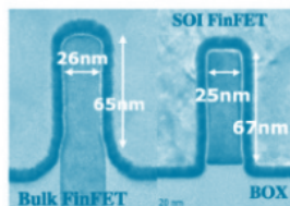
Φωτογραφία ηλεκτρονικού μικροσκοπίου ενός σύγχρονου τρανζίστορ, νέας αρχιτεκτονικής, με πύλη μόλις 25νανόμετρα
